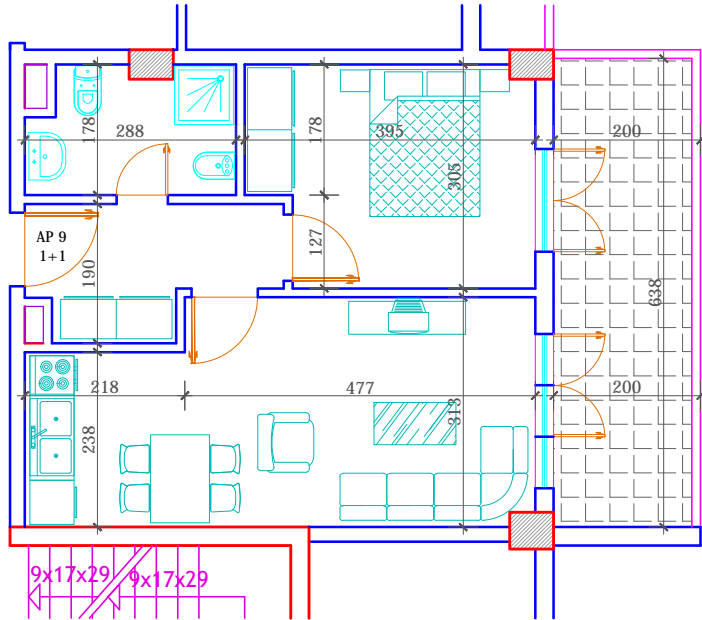
PLANIMETRIA E AP.2/4/9 SH.1:100
