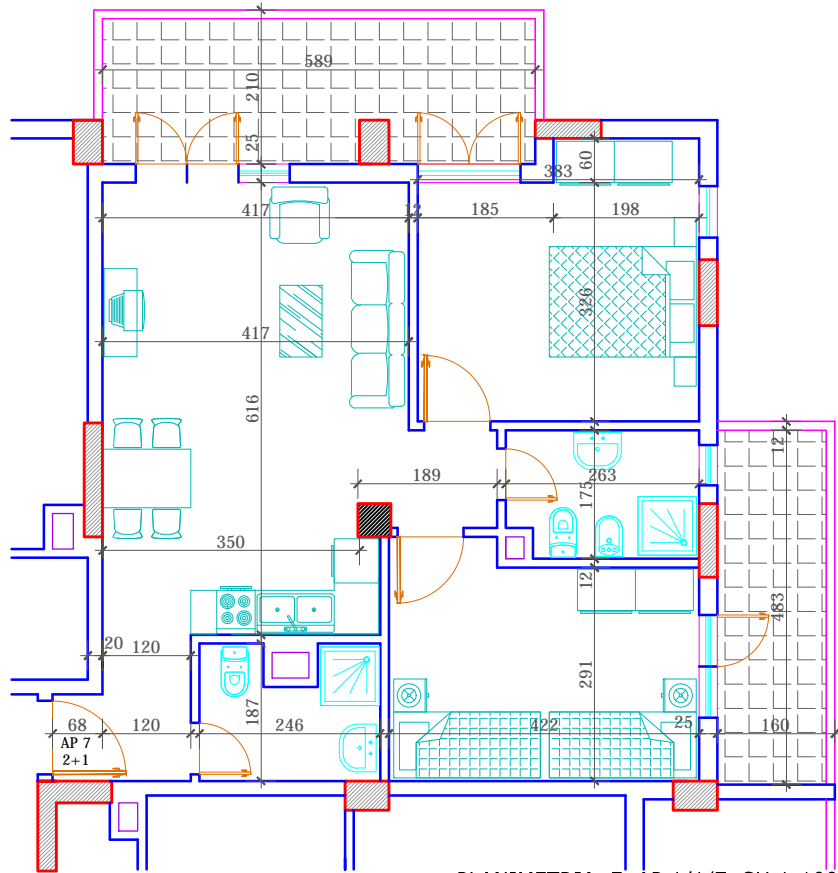
PLANIMETRIA E AP.1/1/7 SH.1:100
