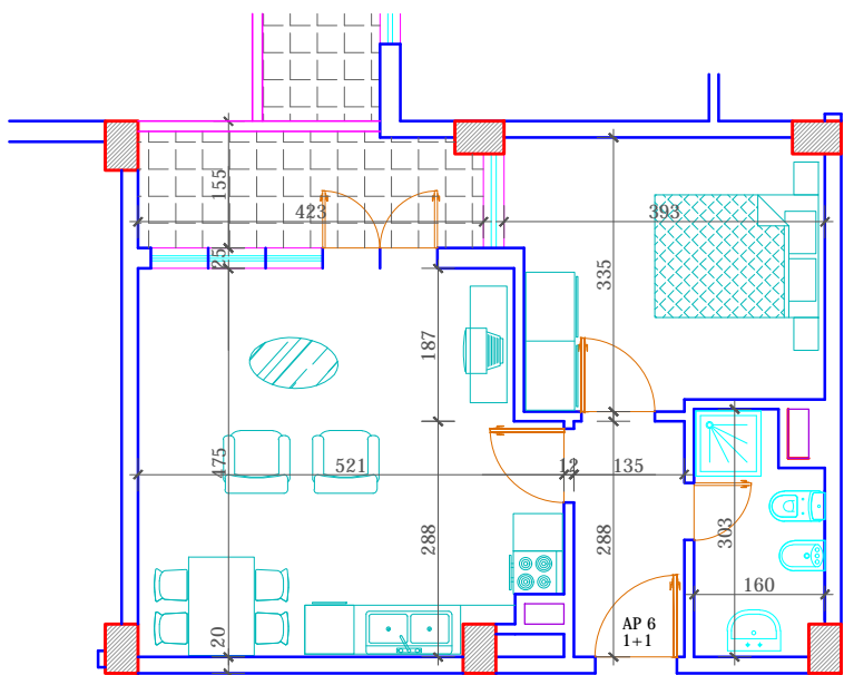
PLANIMETRIA E AP.2/4/6 SH.1:100
