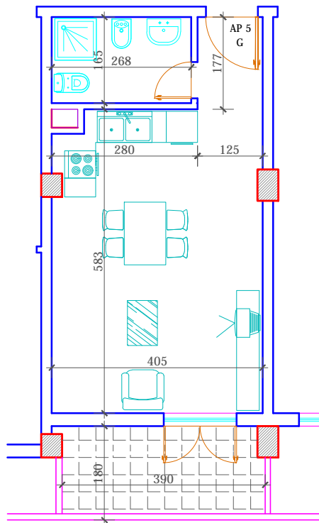
PLANIMETRIA E AP.2/1/5 SH.1:100
