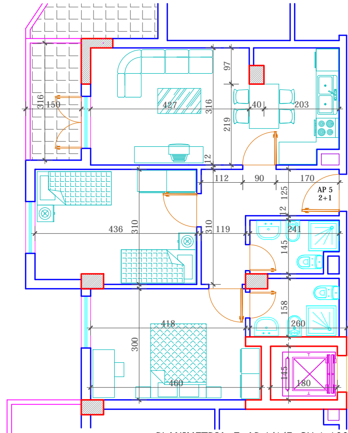
PLANIMETRIA E AP.1/1/5 SH.1:100
