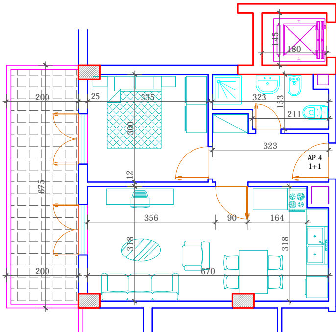
PLANIMETRIA E AP.1/1/4 SH.1:100
