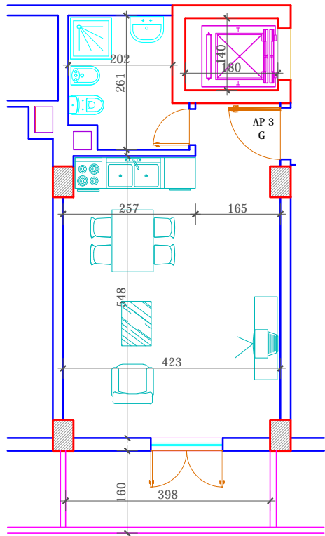
PLANIMETRIA E AP.2/4/3 SH.1:100
