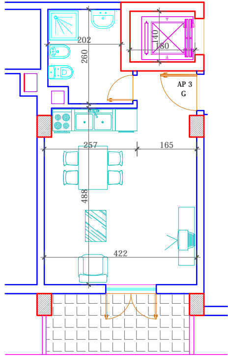
PLANIMETRIA E AP.2/1/3 SH.1:100
