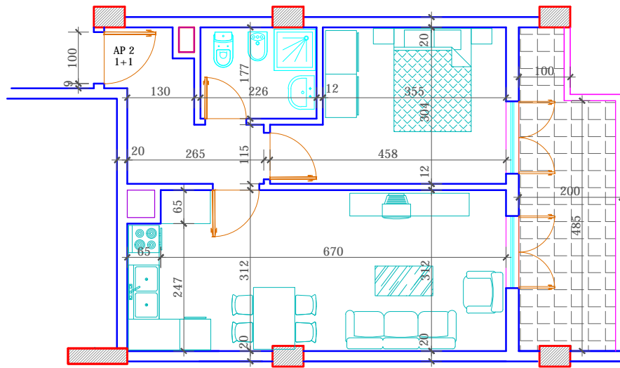
PLANIMETRIA E AP.1/1/2 SH.1:100
