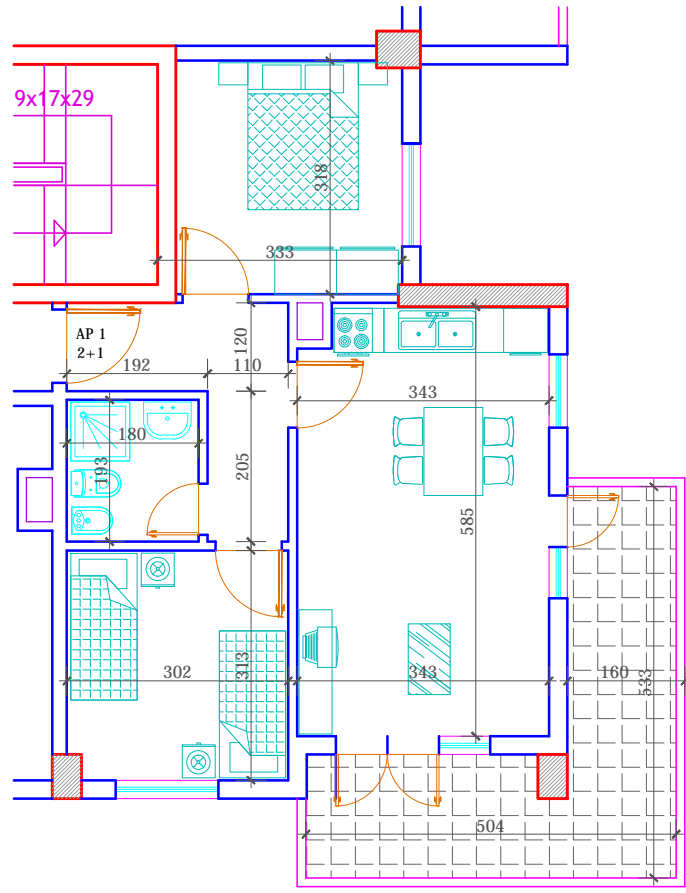
PLANIMETRIA E AP.2/4/1 SH.1:100
