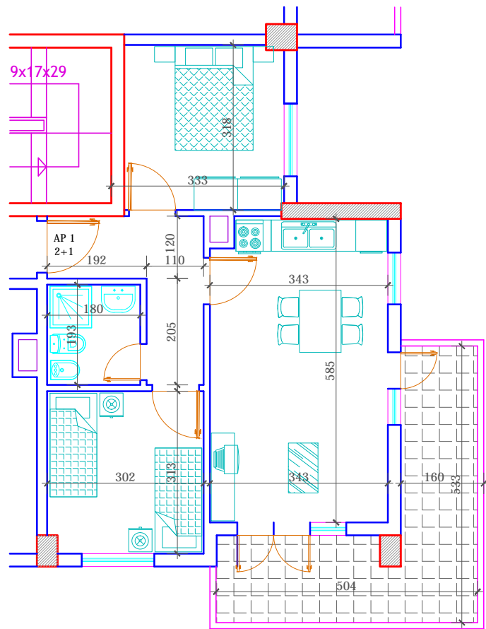
PLANIMETRIA E AP.2/1/1 SH.1:100
