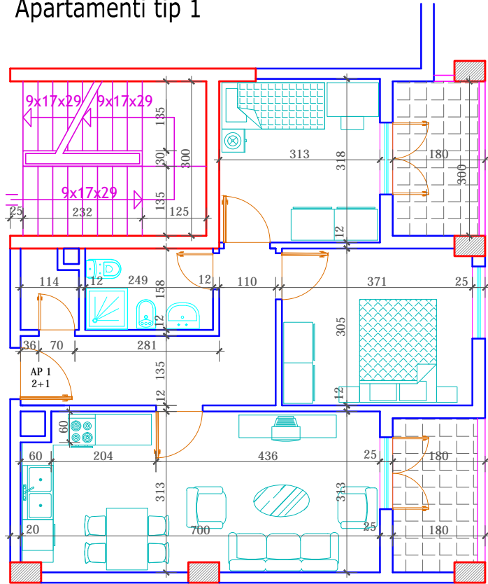
PLANIMETRIA E AP.1/1/1 SH.1:100
